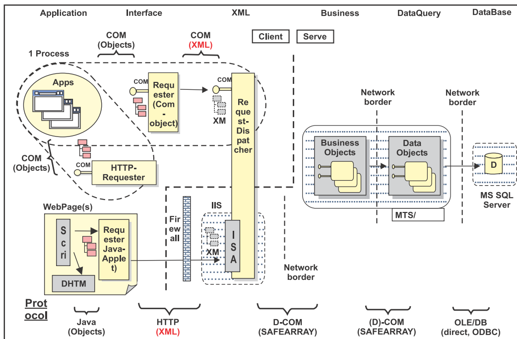
Ενδεικτική αρχιτεκτονική υλοποίησης ενός ΣΔΕ
