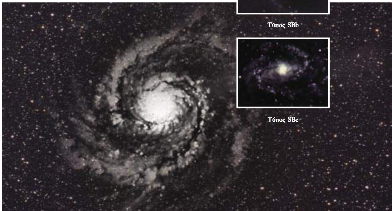
Σπειροειδής γαλαξίας NGC1365. Οι φωτεινοί του βραχίονες ξεκινούν από μία κεντρική ράβδο.
